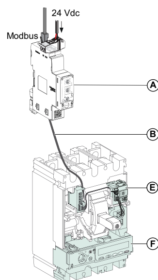
Ejemplo 4: Conexión de la interfaz de comunicación IFM al módulo BSCM Modbus SL/ULP y a la unidad de control MicroLogic 5, 6 o 7
