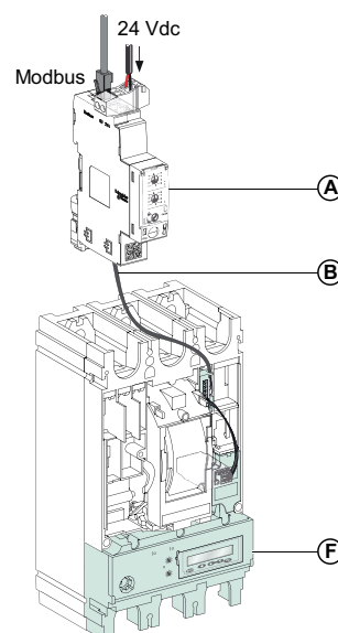
Ejemplo 2: Conexión de la interfaz de comunicación IFM a la unidad de control MicroLogic 5, 6 o 7
